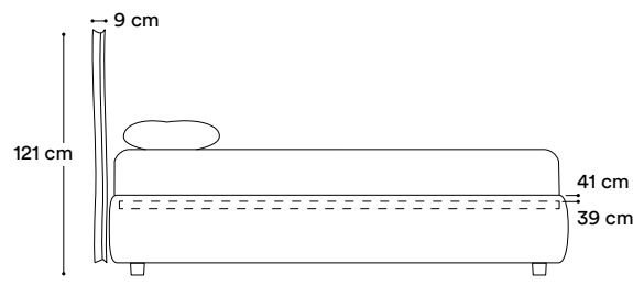
Dimensione esterna / External dimension 207 - 217 cm
